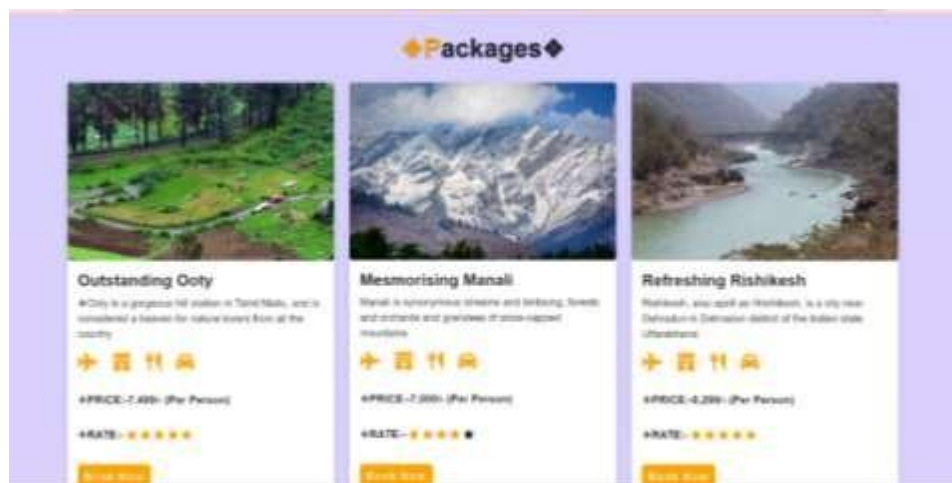
Fig 3.4.2 Packages.
