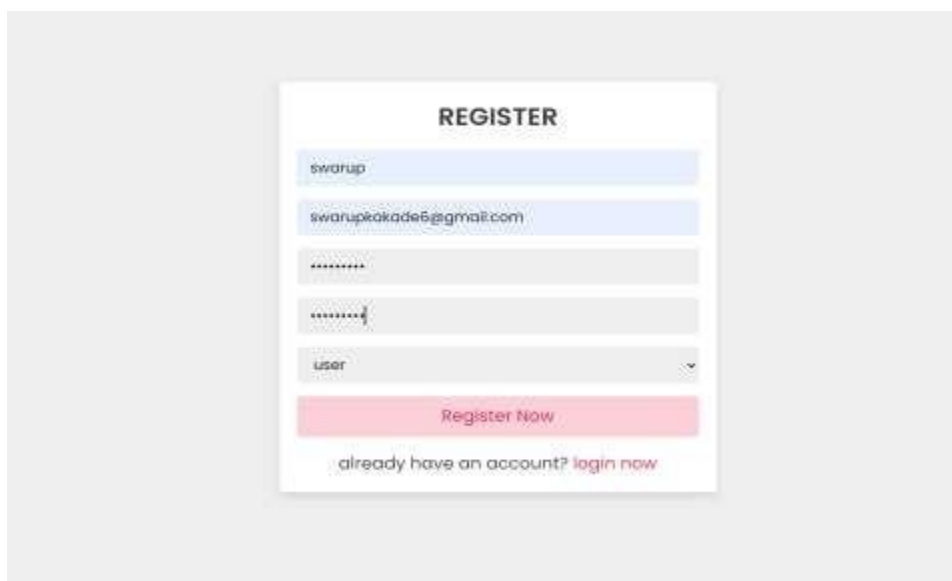
Fig 3.4.3 Registration page.
